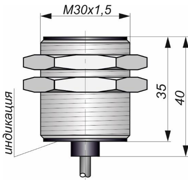
Габаритный чертеж
